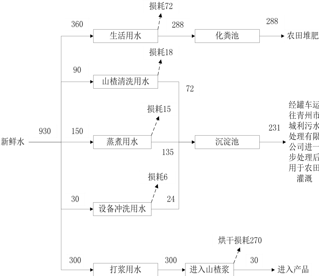
图 2.2-2 项目水量平衡图 单位： \text{m}^3/\text{a}
