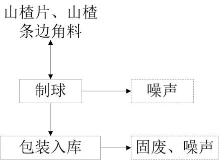
图 2.3-2 山楂球生产工艺流程及产污环节图
