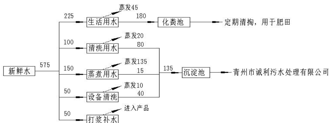
图 2.2-2 项目水量平衡图
