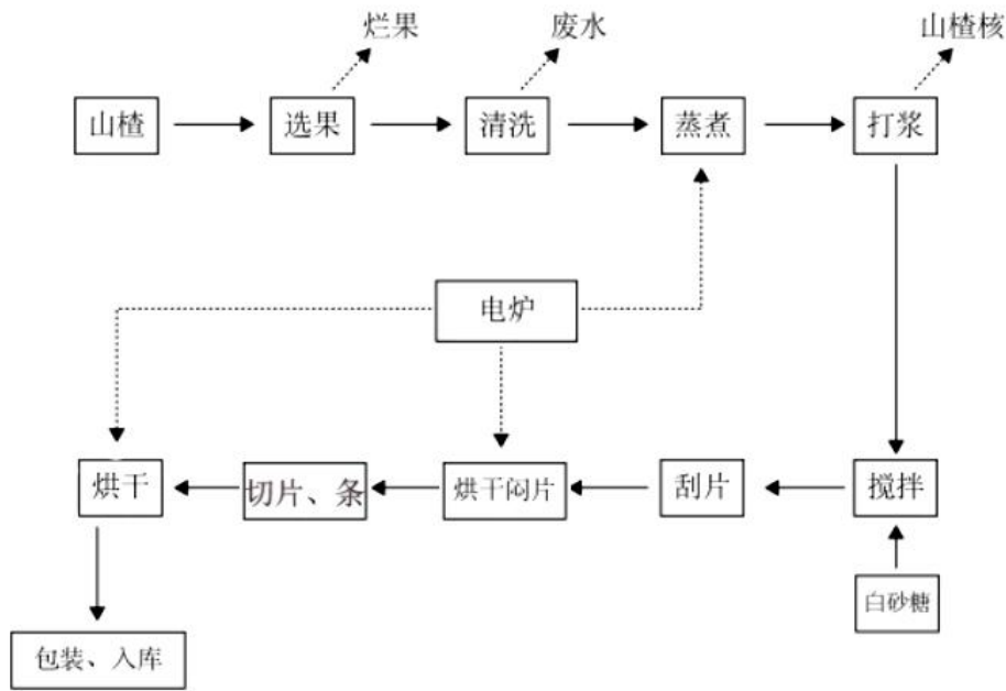
图 2.3-1 工艺流程及产污环节示意图
