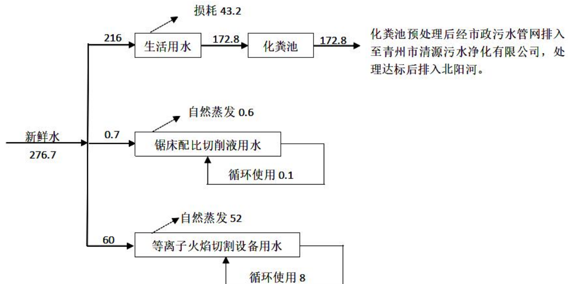
图 2.2-1 项目水平衡图 (单位 m³/a)
